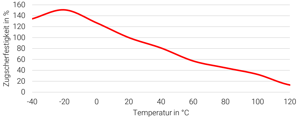
Zugscherfestigkeit bei unterschiedlichen Temperaturen in %
