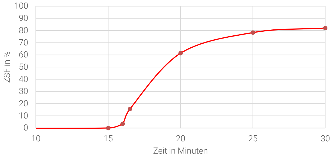
Festigkeitsaufbau Zugscherfestigkeit in %
