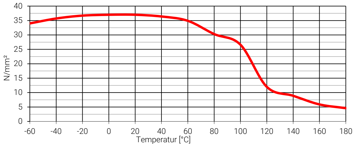
Abb. 1: Zugscherfestigkeit vs. Temperatur Stahl-Stahl-Verklebung; 100% = Festigkeit bei 23 °C.
